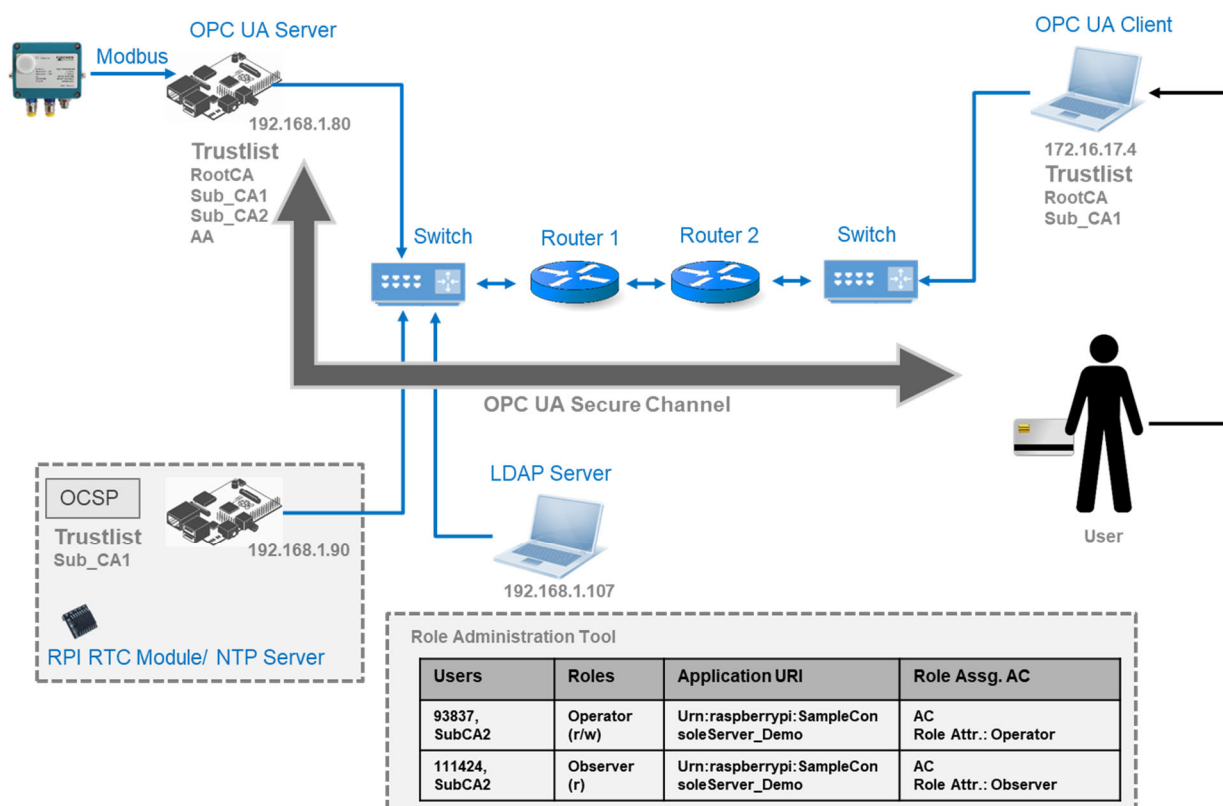
Abbildung 29: OPC UA sicherer Verbindungsaufbau
