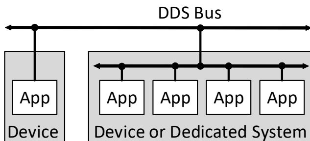
Abbildung 7: DDS-Architektur in einem Edge-Netzwerk mit Edge-Geräten
