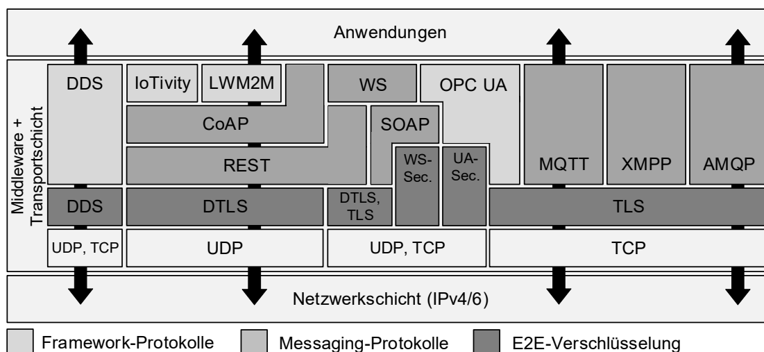
Abbildung 24: Strukturiertes Modell der evaluierten Middleware-Protokolle
