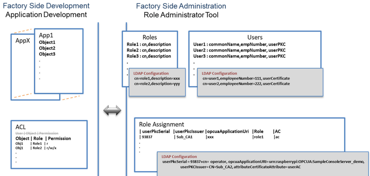
Abbildung 26: Einsatzumgebungen des Role Administration Tools
