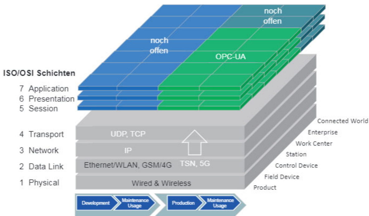
Abbildung 12: Gegenwärtige Festlegungen im Communication Layer [72]
