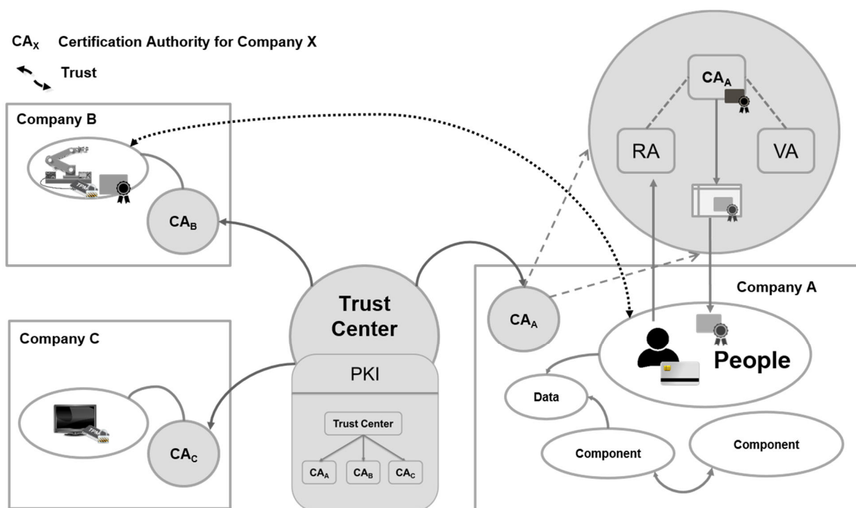
Abbildung 18: Sichere Ende-zu-Ende-Kommunikation innerhalb und über Unternehmensgrenzen hinweg [100]
