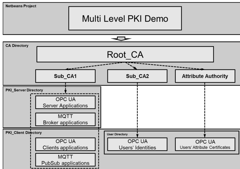
Abbildung 23: Multilevel PKI für den Demonstrator
