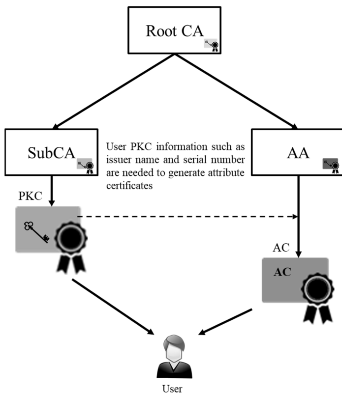
Abbildung 21: PKI und Attribute Authority [24]
