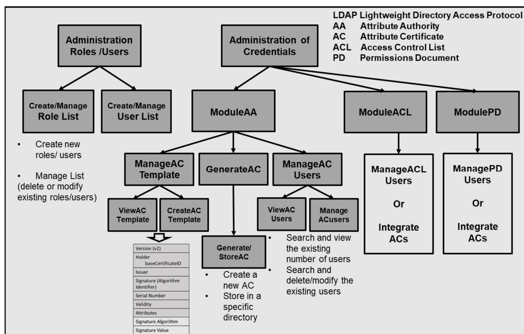
Abbildung 25: Role Administration Tool – Wesentliche Module
