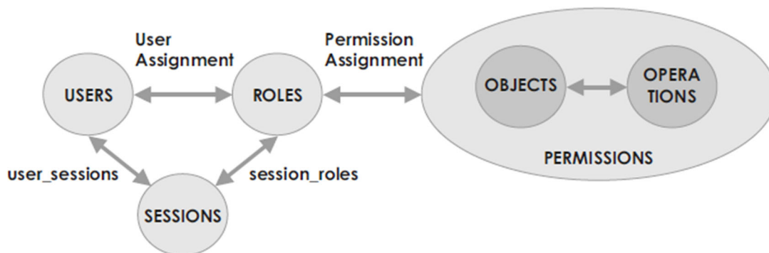
Abbildung 17: RBAC-Konzept [91]
