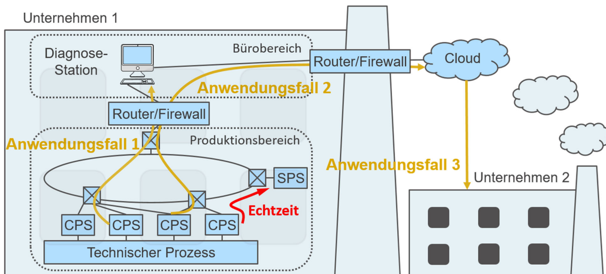
Abbildung 16: Anwendungsfälle 1-3
