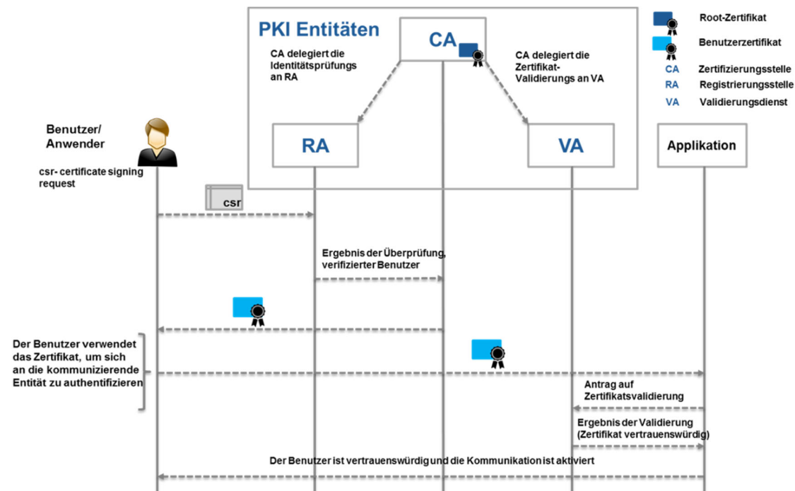
Abbildung 3: Einfache Public-Key-Infrastruktur
