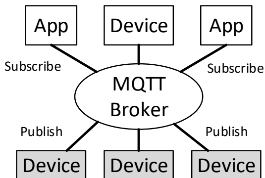
Abbildung 4: MQTT Pub/Sub-Architektur
