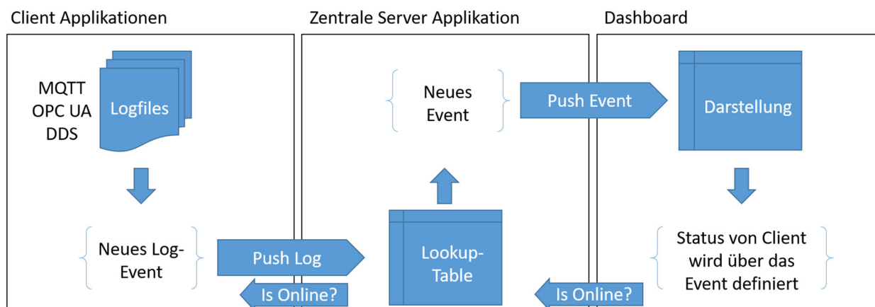
Abbildung 27: Monitoring-Tool
