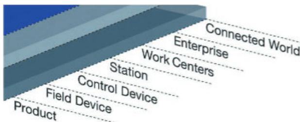
Abbildung 10: Hierarchie-Achse [72]
