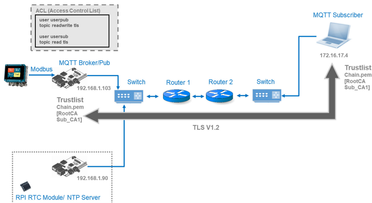
Abbildung 30: MQTT sicherer Verbindungsaufbau
